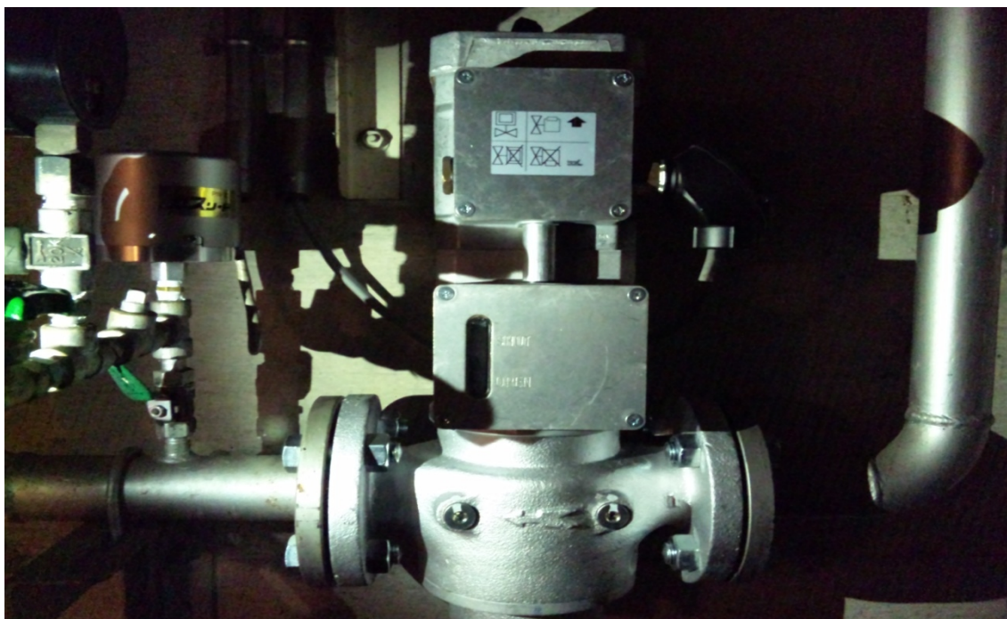
遮断装置 HK1 (CKD 社) / 圧カスイッチ PN-2 (GSE 社)
